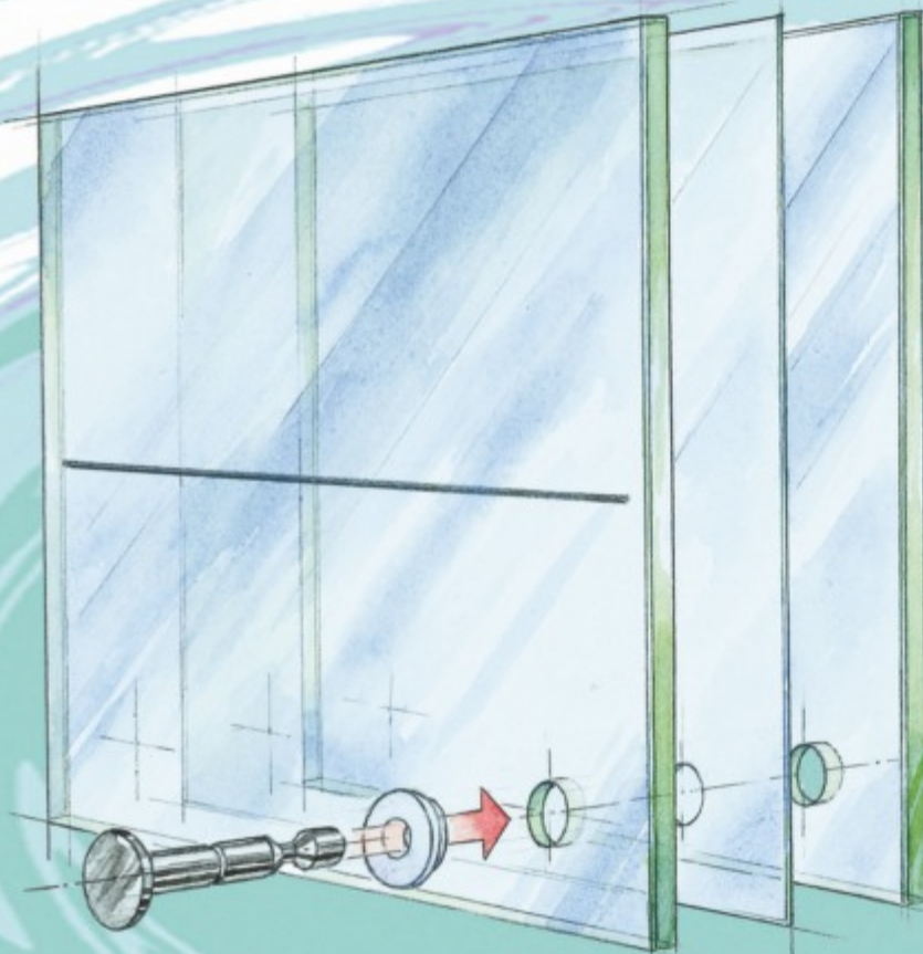
Denne tegning viser tydeligt sandwich-konstruktionen af glas og rustfrit stål beslag.
